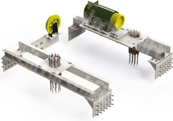
DIŞLİSİZ MAKİNA ŞASESİ GEARLESS MOTOR STAND
